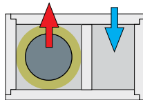
Abgas- und separater Zuluftschacht. Für raumluftunabhängige Festbrennstofföfen
