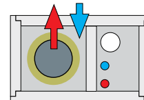
Abgas- und Zuluft- und separater Installationsschacht. Für raumluftunabhängige Festbrennstofföfen und Haustechnik
